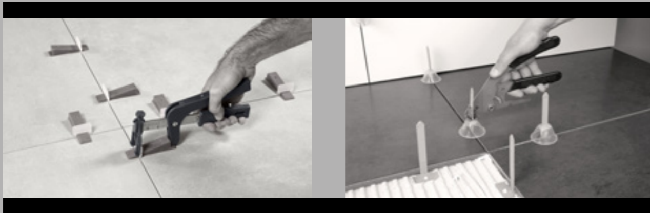
A LEVELING SYSTEM BY RAIMONDI SISTEMA DE NIVELACIÓN RAIMONDI
