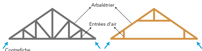
Figure 2 : Schéma de fermette de type « en N » en métal (gauche) et de type « à entrain retourné » en bois (droite)
